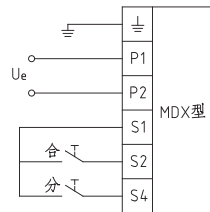
MDX 型电动操作机构接线图
